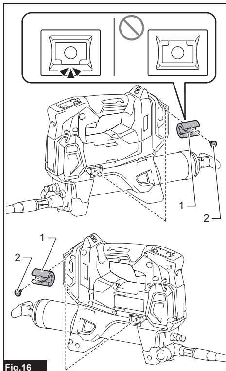
► 1. Support de tuyau 2. Vis
